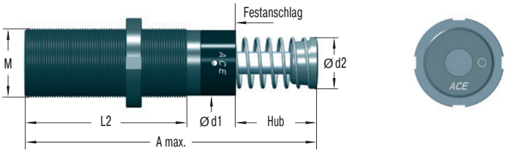
Gewinde M36x1,5 und M42x1,5 auf Anfrage Gewinde UNF 1 1/4-12 (Bestellbezeichnung ohne Endung M)
