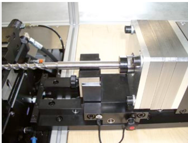
Les bloqueurs d'ACE jouent leur rôle dans la production d'outils de perçage : le système LOCKED-P bloque, tout en absorbant sans difficulté les forces opposées du processus d'assemblage GRAF automation GmbH, 88214 Ravensburg, Allemagne
