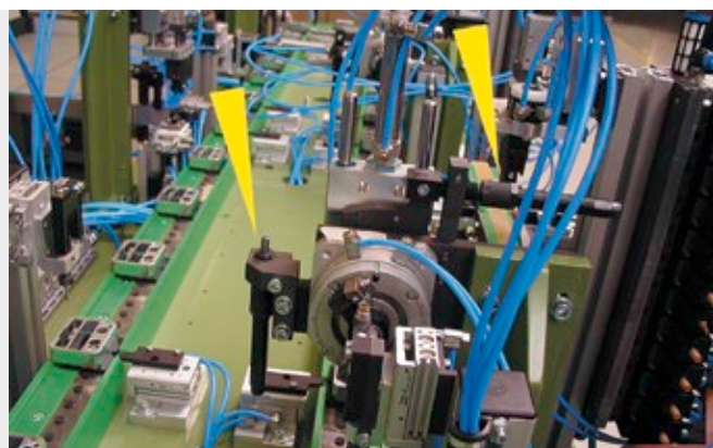
Production optimisée dans l'industrie électronique Stebie Maschinenbau GmbH, Allemagne
