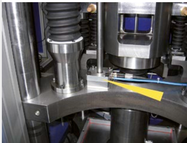
Le blocage de tige pneumatique permet d'utiliser des presses hydrauliques pour toute application KOMAGE Gellner Maschinenfabrik KG, 54427 Kell am See, Allemagne
