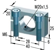
MB20 Bloc de bridage
