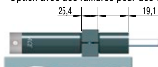
Montage pour VC25...F avec KB... (23,8 mm sans filetage)
