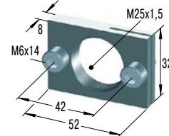
RF25 Rechteckflansch
