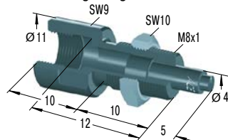
BV8A Bolzenvorlagerung
