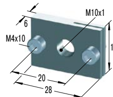
RF10 Rechteckflansch
