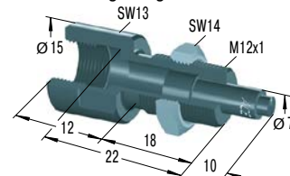
BV12SC Bolzenvorlagerung
