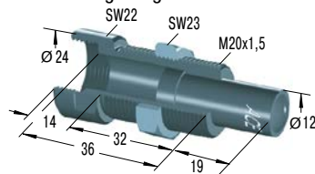
BV20SC Bolzenvorlagerung
