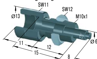
BV10SC Bolzenvorlagerung
