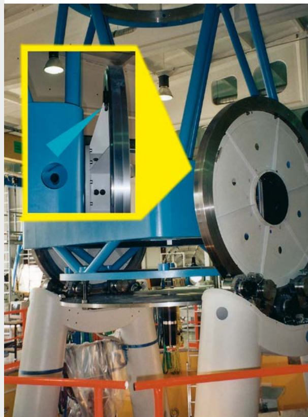
Perfekter Überfahrtschutz für Präzisionsteleskop
