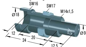
BV14 Bolzenvorlagerung
