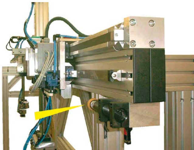
Industriestoßdämpfer optimieren am Portal
