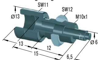
BV10 Bolzenvorlagerung
