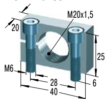
MB20 Klemmflansch
